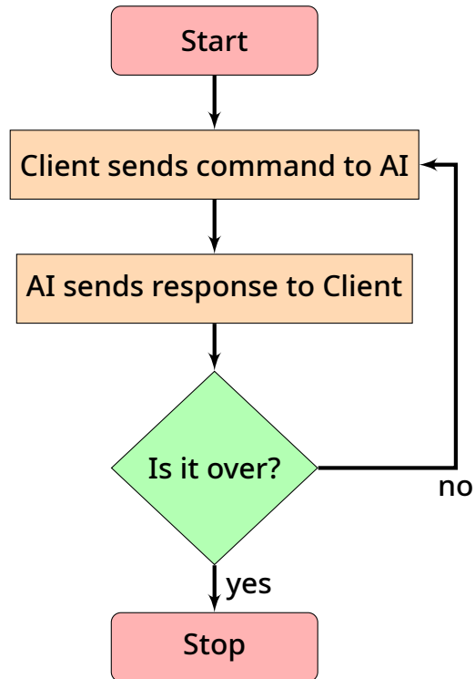
Figure 21: MGTP 流程圖
